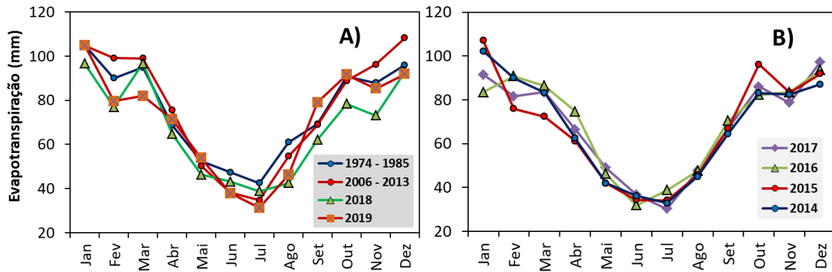
Figura 5: Evapotranspiração potencial mensal (mm mês -1 ) do período de 1974-1985, 2006-2013, 2018 e 2019 (A) e dos anos de 2014, 2015, 2016 e 2017 (B) para a região do Sul de Minas, Muzambinho, MG.
