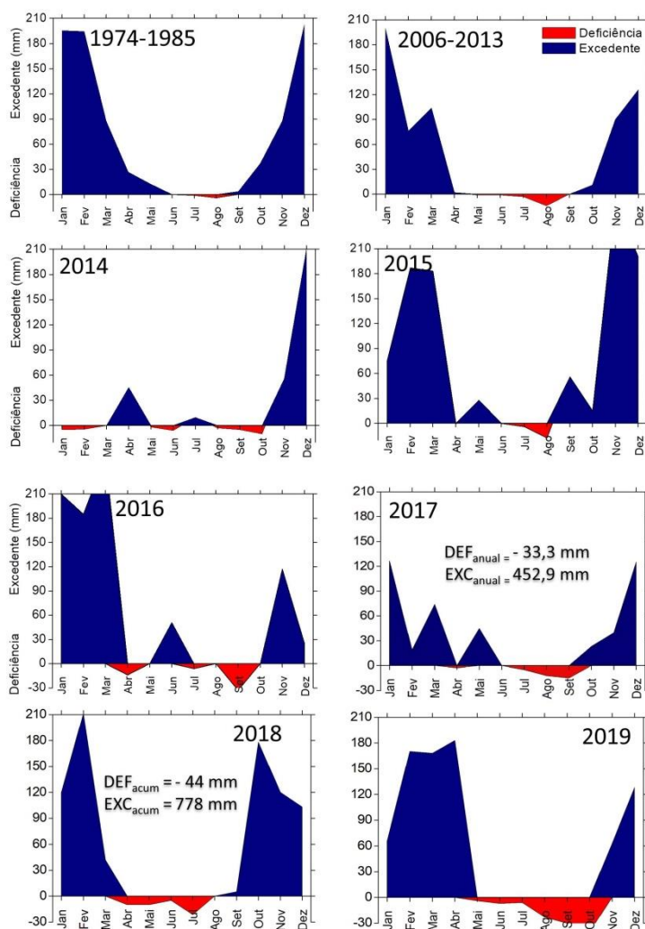
Figura 8: Balanço hídrico mensal sequencial (THORNTHWAITTE E MATHER, 1955) no período de 1974-1985 (A), 2006-2013 (B), para os anos de 2014 (C), 2015 (D), 2016 (E), 2017 (F), 2018 e 2019 para a região do Sul de Minas, Muzambinho.
